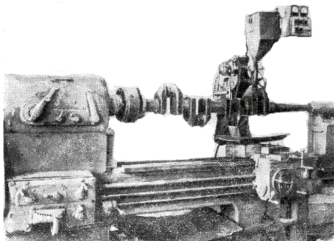
Рис. 5. Токарний верстат, пристосований для наплавлення колінчатих валів під шаром флюсу
